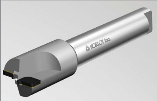
Рассверливание
